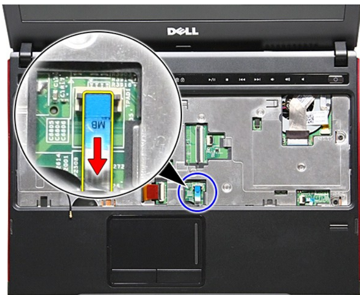
19. ปลดสายทัชแพดออกจากขั้วต่อที่เมนบอร์ด
