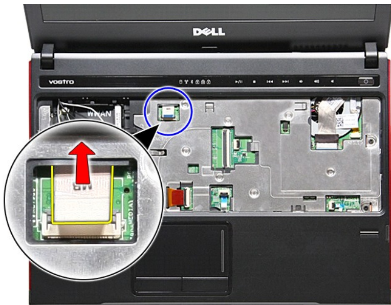
15. ปลดสายป้อนมีเดียจากข้อต่อที่เมนบอร์ด
