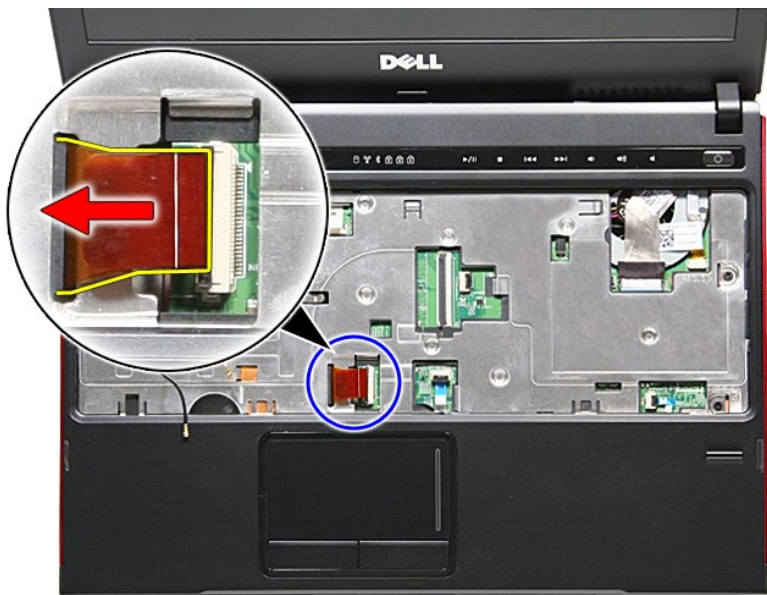
17. ปลดสายข้อมูล ExpressCard ออกจากขั้วต่อที่เมนบอร์ด
